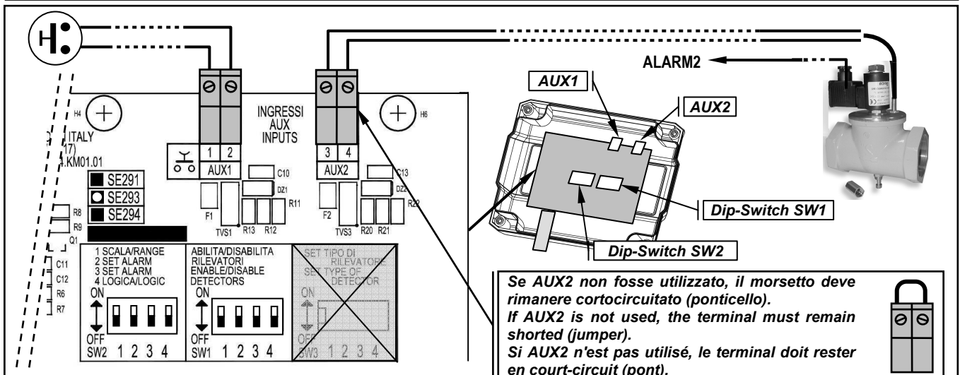
Fig. 7 - AUX1 Collegamento di un Pulsante manuale NA all'ingresso AUX1. / Wiring diagram, of a NO manual button at the AUX1 input / Schéma avec un bouton manuel NF à l'entrée AUX1
