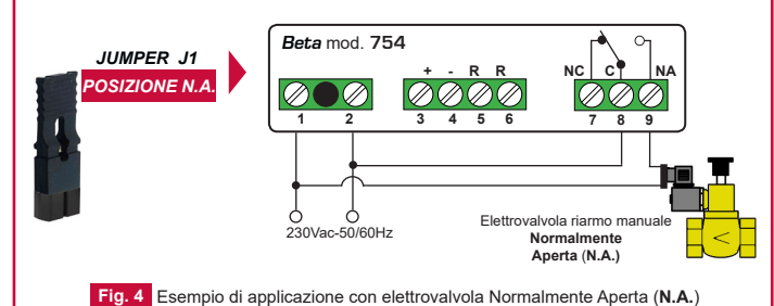
Fig. 4 Esempio di applicazione con elettrovalvola Normalmente Aperta (N.A.)
