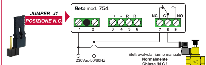
Fig. 5 Esempio di applicazione con elettrovalvola Normalmente Chiusa (N.C.)
